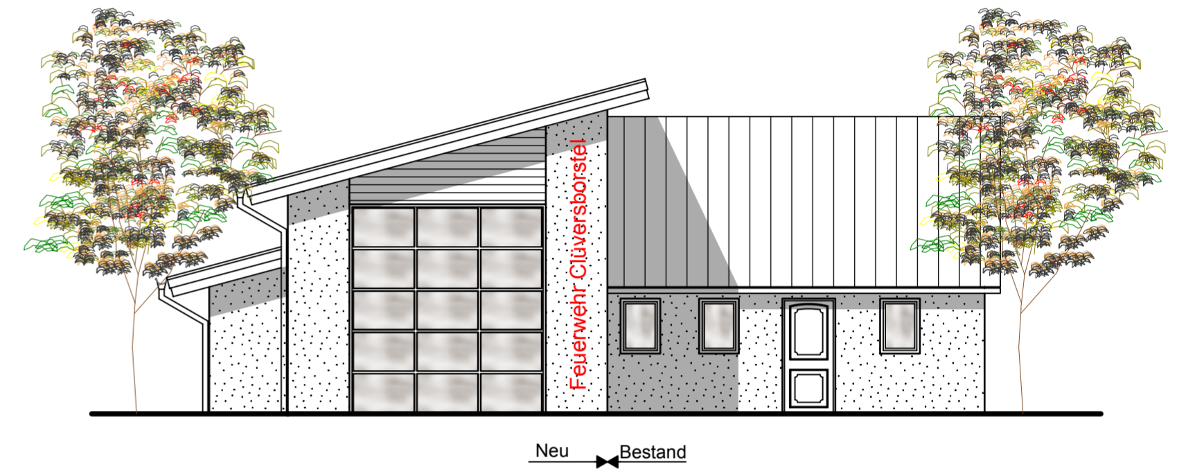
Ansicht Süd
